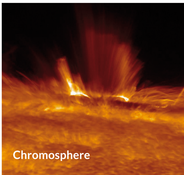
Fibrils
